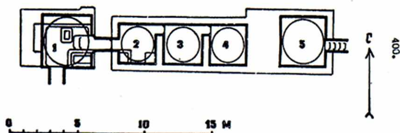
Манзара. Тарҳи Ҳаммом.
