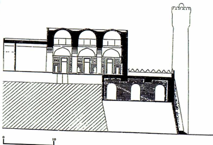
Ҳулбук. Масҷиди қаср.
